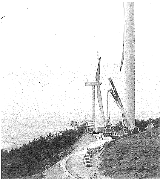
Montaje del parque con el valle del Ebro al fondo. s.n.
